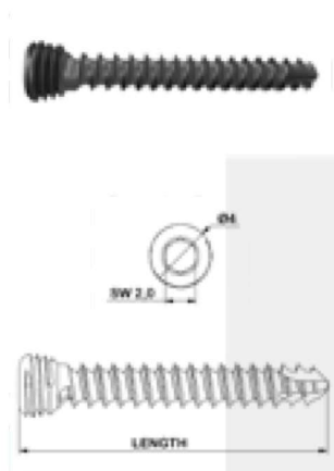
2.4 mm Mini Locking Screw
