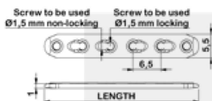
1.5 mm Mini Straight Compression Locking Plate
