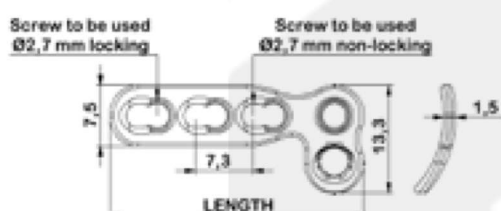
2.7 mm Mini L Locking Plate
