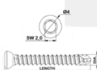
2.4 mm Mini Screw
