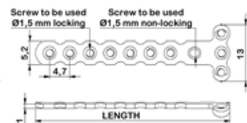
1.5 mm Mini Locking Plate
