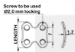
2.0 mm Mini Adaptation Locking Plate
