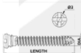
2.0 mm Mini Locking Screw
