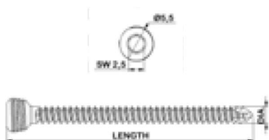
2.7 mm Mini Locking Screw ( 5.5 mm Head DIA. )
