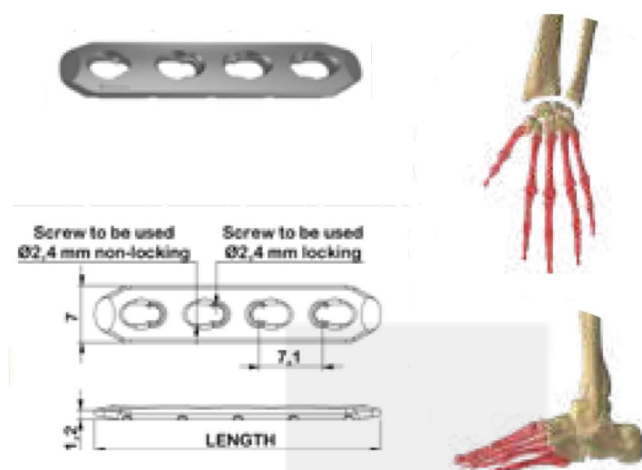
2.4 mm Mini Straight Locking Plate
