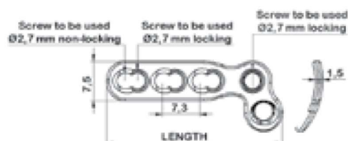
2.0 mm Mini Oblique L Locking Plate
