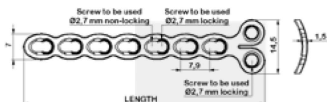
2.7 mm Mini Condylar Locking Plate
