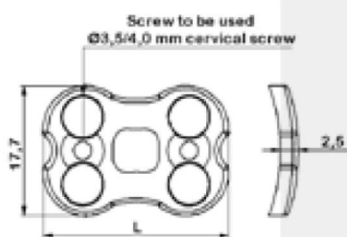
Anterior Cervical Plate 1
